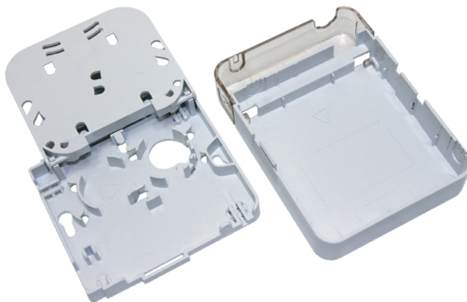
Рисунок 2 - Внутренний конструктив
